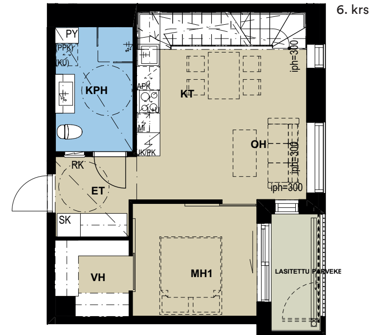
Ullakkokerros
